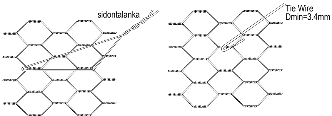
Kuva 8 – Asennus ja täyttö – Kivikorit – Tukilangat käyttäen sidontalankaa tai Tie Wire - sidontalennkkejä
