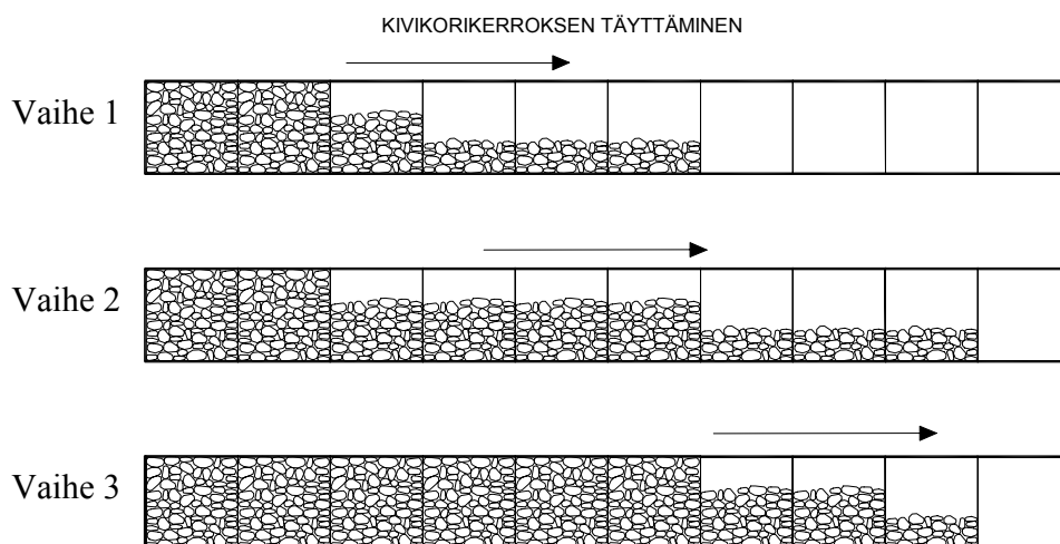
Kuva 6 – Asennus ja täyttö – Kivikorit
