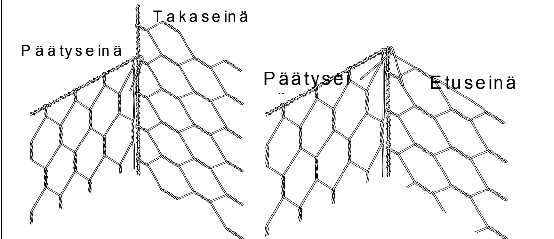
Kuva 3 – Kokoaminen - Kivikorit – Liitokset päätyseinien ja etu/takaseinien reunakohtissa
