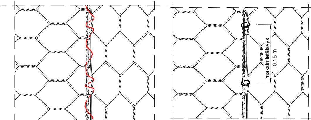
Kuva 5 – Saumakohtien kiinnitys – Liitokset käyttäen sidontalankaa tai Spenax-renkaita
