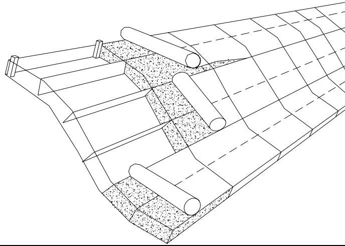
Kuva 11 – Asennus ja täyttö – Reno Mattressit – Kannen asennus luiskan suuntaisesti
