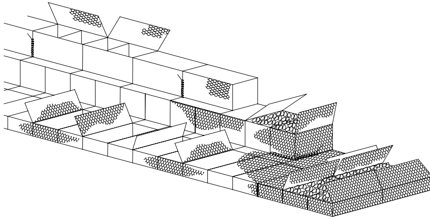
Kuva 7 – Asennus ja täyttö – Kivikorit
