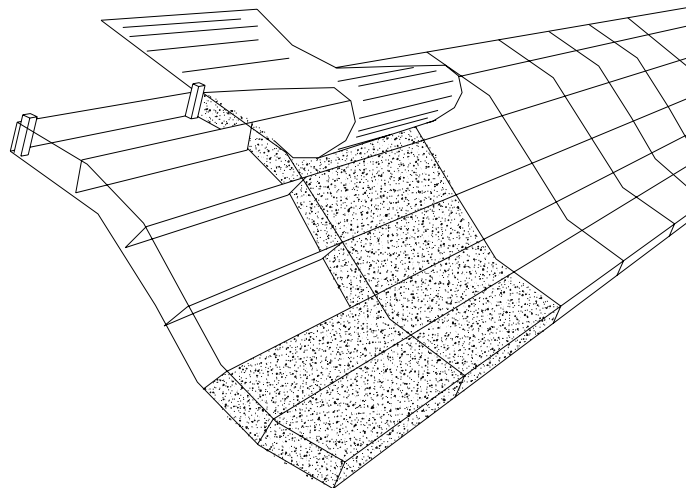
Kuva 10 – Asennus ja täyttö – Reno Mattressit – Kannen asennus Mattressien suuntaisesti
