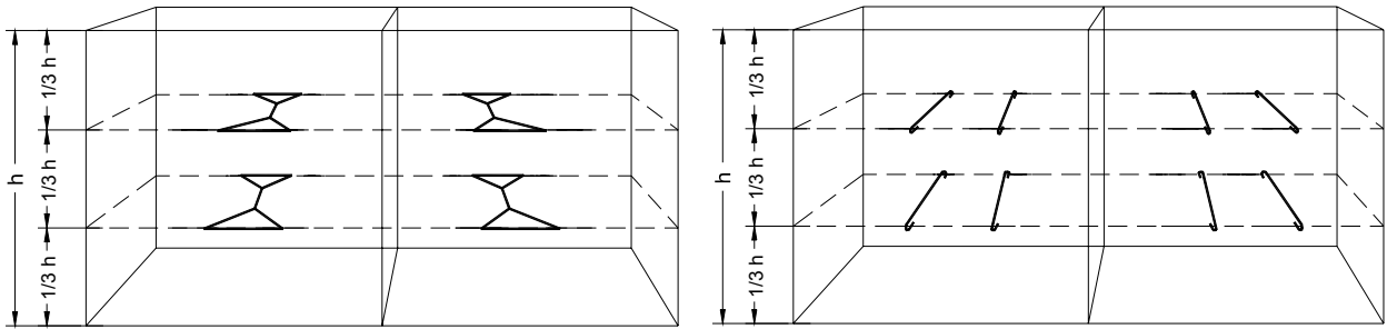
Kuva 9 – Asennus ja täyttö – Kivikorit – Tukilangat
